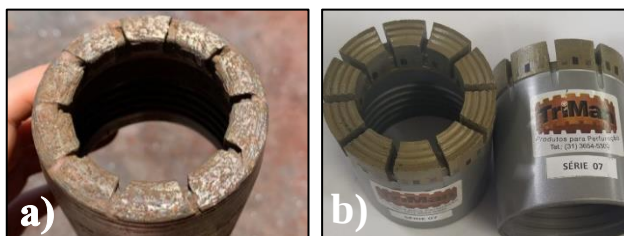
Figura 2 – A) 30356 série 07 usada. B) Coroa idêntica a 30356, sem uso.
